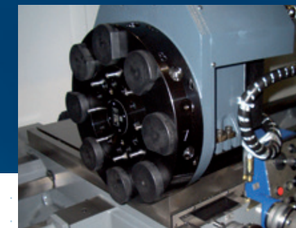
8-fach-Scheibenrevolver mit angetriebenen Werkzeugen, Schaft-ø 40 mm
