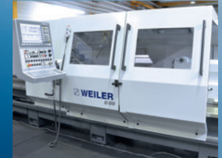
Ausführung mit zweiter Schiebeschutzhülle und Spritzwand
