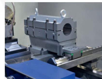
Bohrbock mit zusätzlicher Abstützung
