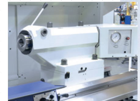
Reitstockpinole hydraulisch betätigt
