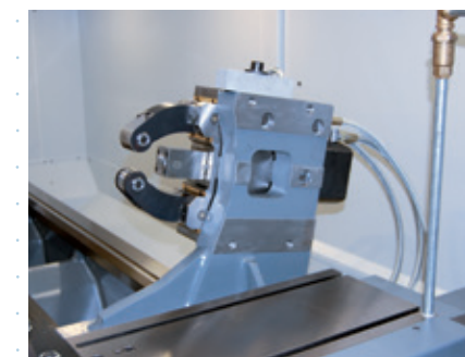
Mitlaufende, selbstzentrierende Lünette, hydraulisch betätigt
