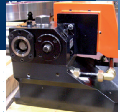
Werkzeugträgerkopf mit angetriebenen Werkzeugen, Aufnahme Capto C8
