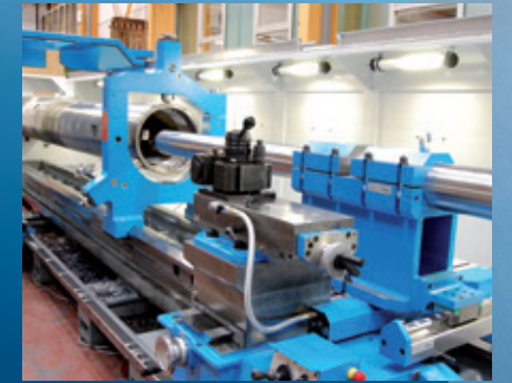
Verstärkter Bohrbock mit zusätzlicher Abstützung und Aufnahmebohrung 160 mm
