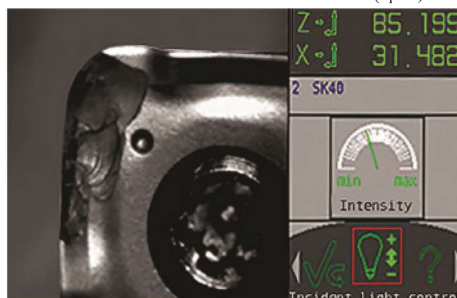
Snijkantsinspectie 12-voudige vergroting van de snijkant in oplicht voor kwaliteitscontrole (optie)
