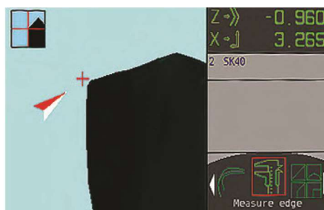
Kompaspijl voor eenvoudig positioneren van de camera voor het meten van nominale maten (optie)
